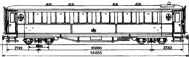
Typenskizze RhB/Club 1889
