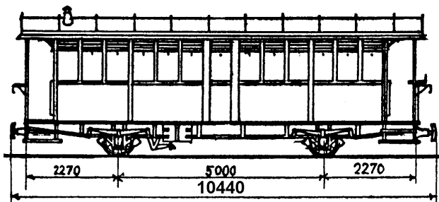
Typenskizze RhB/Club 1889
