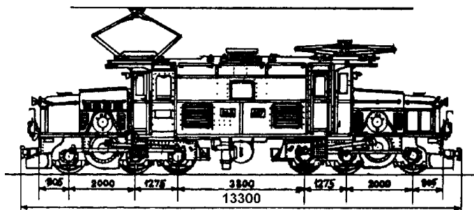
Typenskizze RhB/Club 1889
