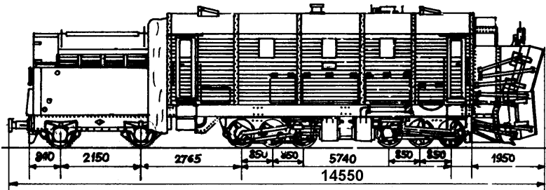
Typenskizze RhB/Club 1889
