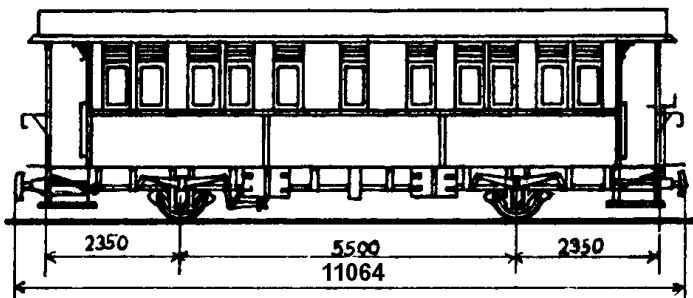
Typenskizze RhB/Club 1889
