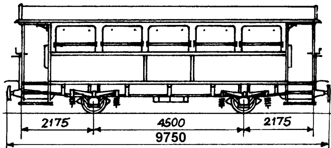
Typenskizze RhB/Club 1889
