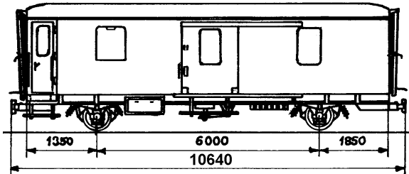
Typenskizze RhB/Club 1889
