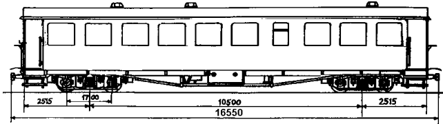
Typenskizze RhB/Club 1889
